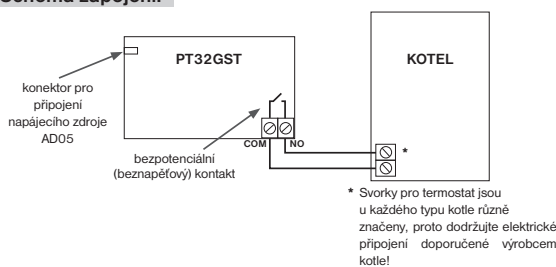
Schéma zapojení:
